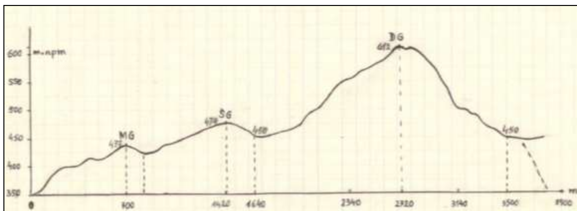
Rys. 3. Grojec – schemat panoramy z zach. Przekrój pasemka góry na linii pn – pd, MG = Mały Grojec; ŚG = Średni Grojec; DG = Duży Grojec
