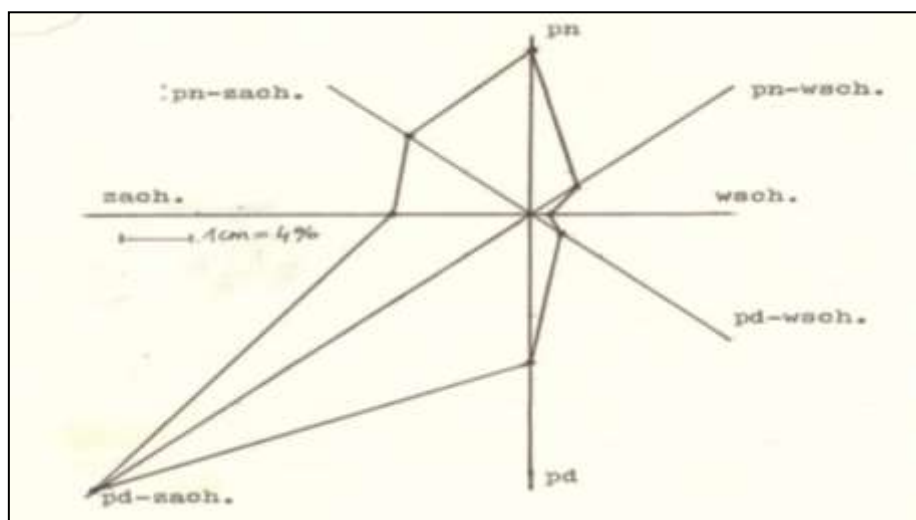
Rys. 11. Rozkład kierunków wiatrów – stacja Porąbka 1961-1970 (wg B. Huczek 1981)
