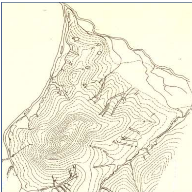
Rys. 7. Mapka Grojca – rzeźba terenu – (poziomice co 20 m.).
