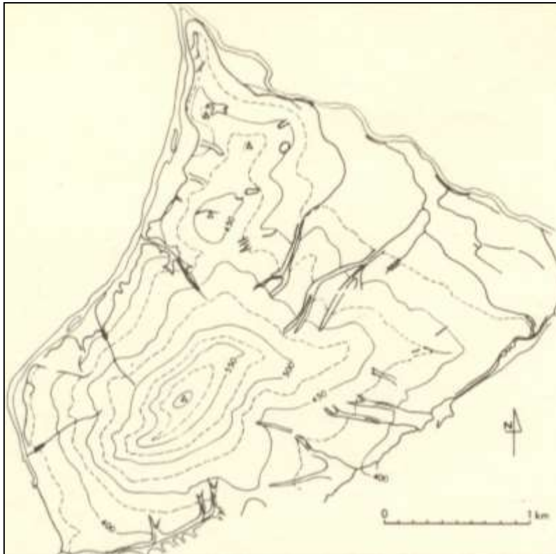
Rys. 6. Mapka Grojca – erozja terenu sływem wód opadowych i gruntowych – (poziomice co 25 m).
