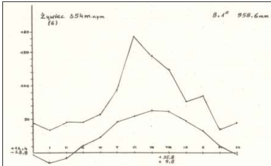
Rys. 13. Klimadiagram dla stacji Żywiec
