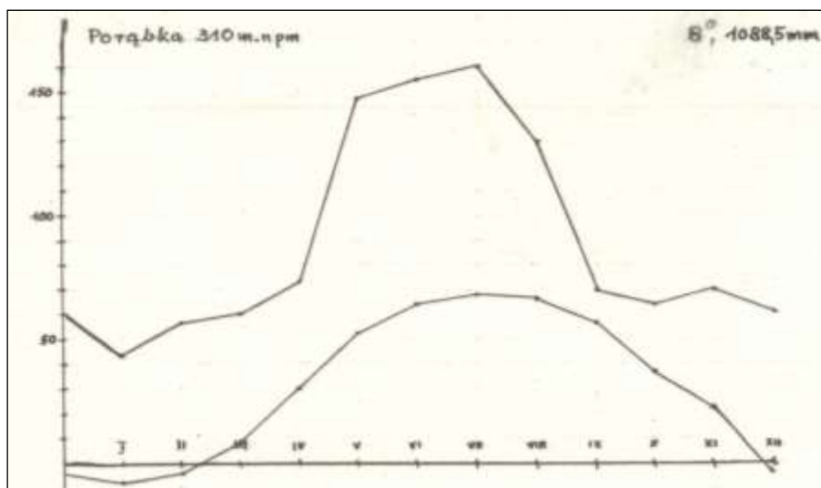
Rys. 12. Klimadiagram dla stacji Porąbka
